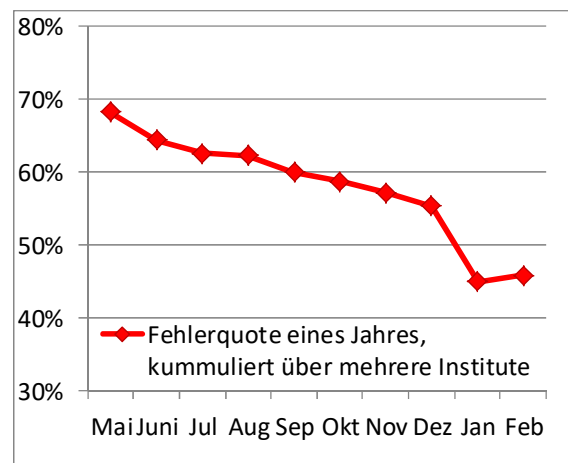
Abbildung 12 "Fehlerquote Alt-Anwender"
