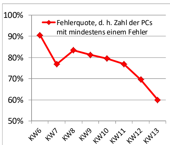
Abbildung 11 "Fehlerquote Erst-Anwender"
