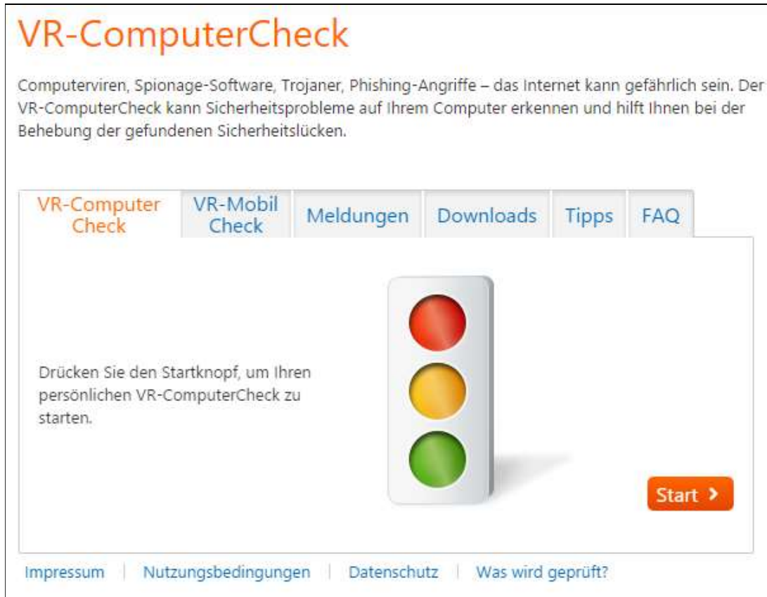
Abbildung 1 "VR-ComputerCheck – „Start-Seite“"
