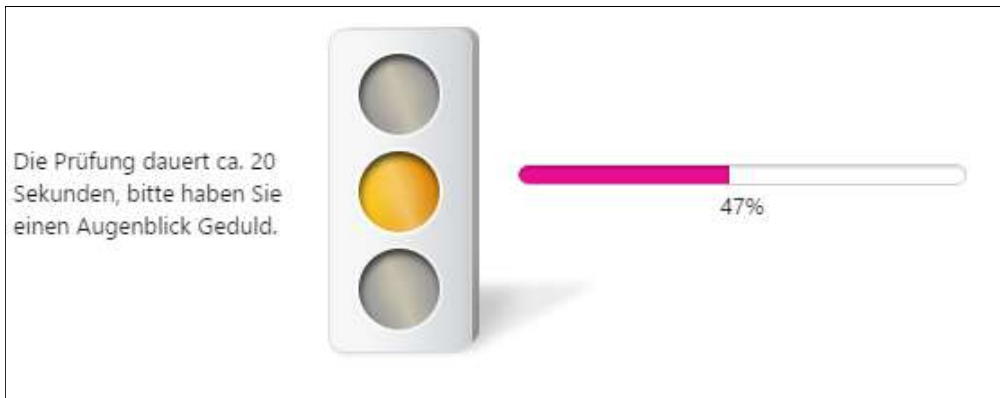
Abbildung 2 "Computercheck – „Läuft-Seite“
