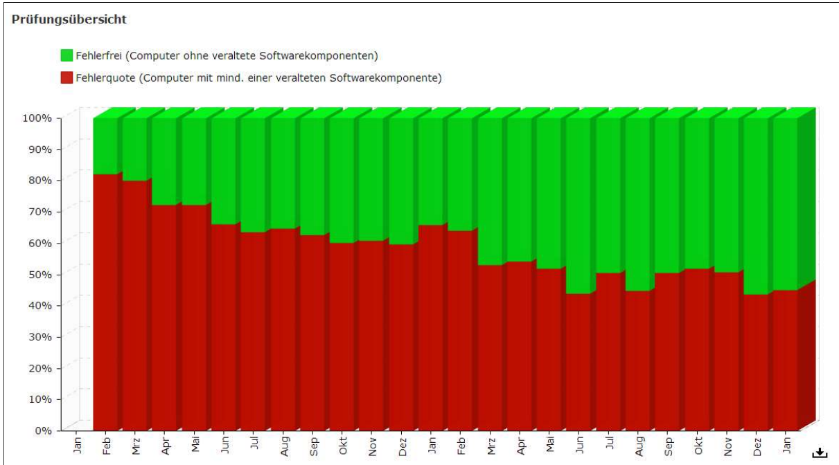
Abbildung 12 "Statistik – Fehlerquote"
